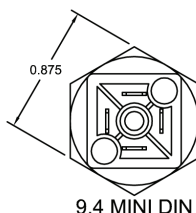
9.4 MINI DIN
